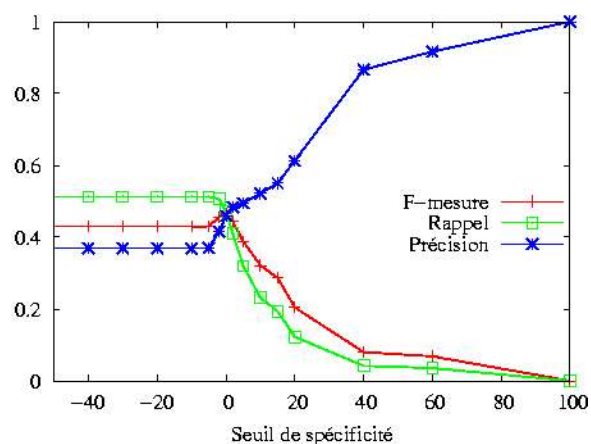
Figure 2: Expérience 2 : variation de R, P et f selon le seuil de spécificité
