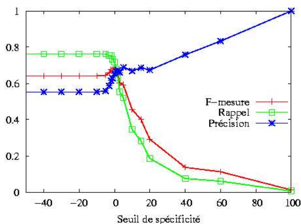
Figure 1: Expérience 1 : variation de R, P et f selon le seuil de spécificité
